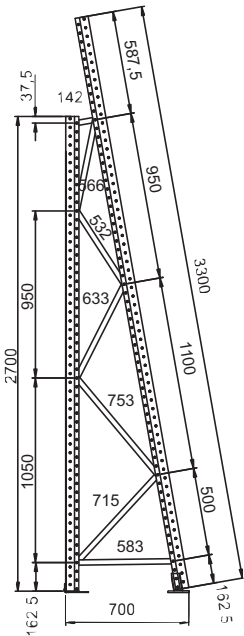
Profillagerregal Einseitig
