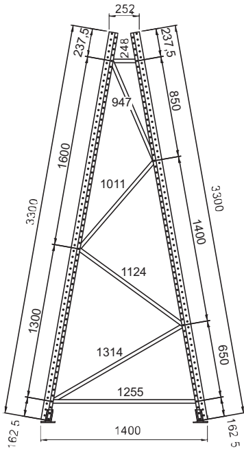
Profillagerregal Zweiseitig
